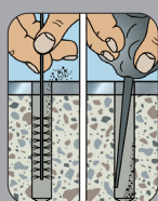
Limpieza del agujero taladrado
